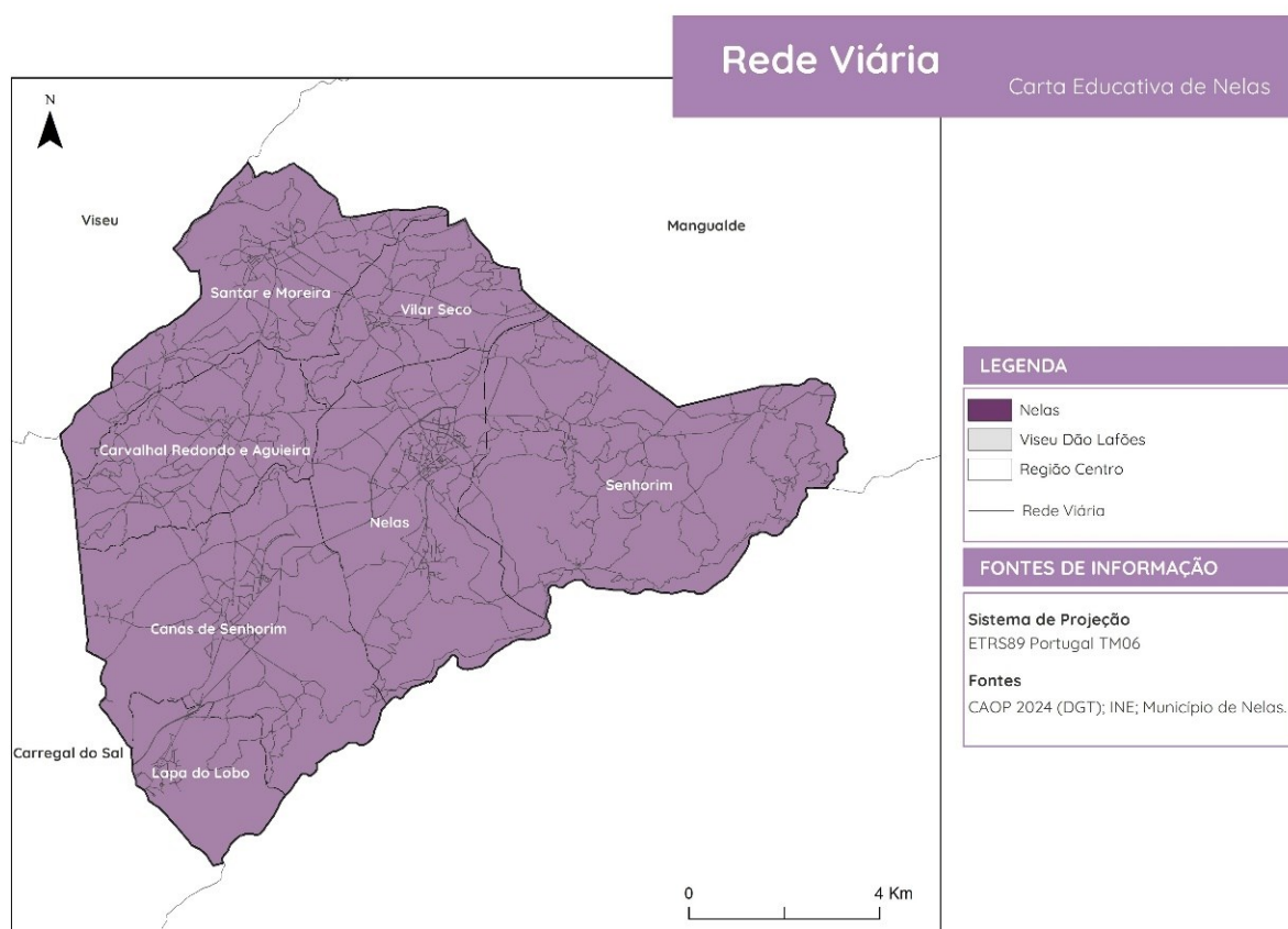
Figura 2. Rede viária de Nelas
